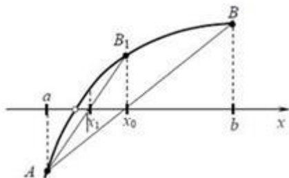
Рис. Построение отрезка (хорды) к функции
