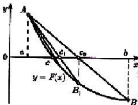
Рис. Пояснение к определению погрешности расчета
