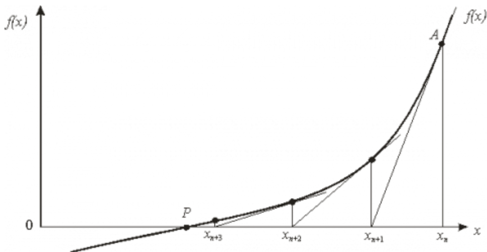
Рис. Графическая интерпретация метода касательных
