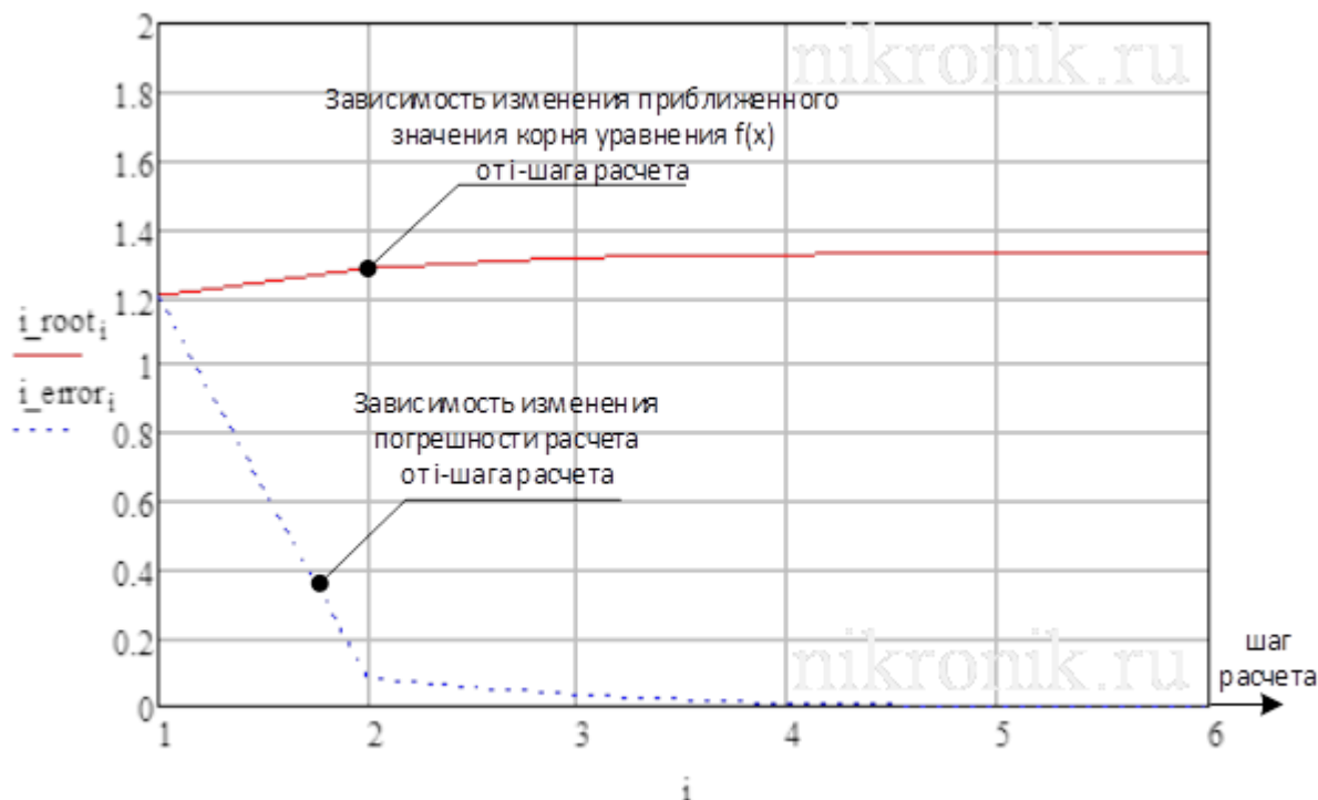
Рис. Результаты расчета по методу хорд
