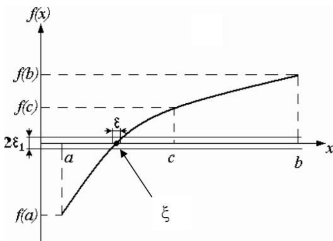
Рис. Графическая интерпретация метода половинного деления
