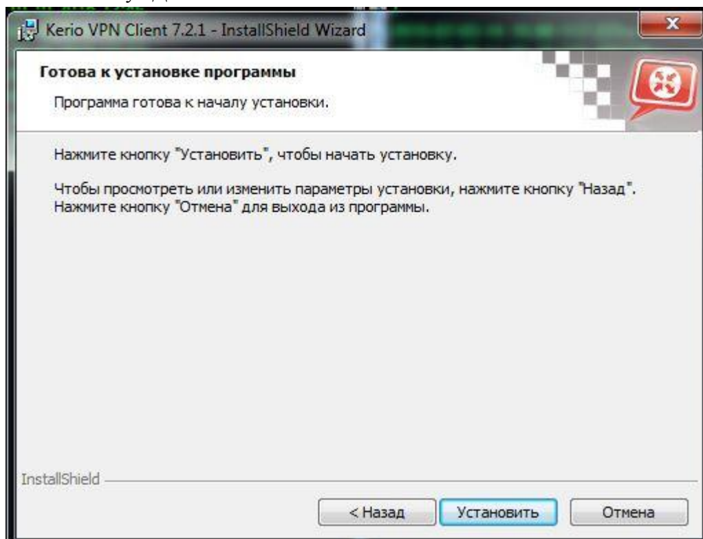
Рис.6. Окно инсталляции
