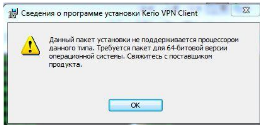
Рис. 3. Сообщение ошибки
